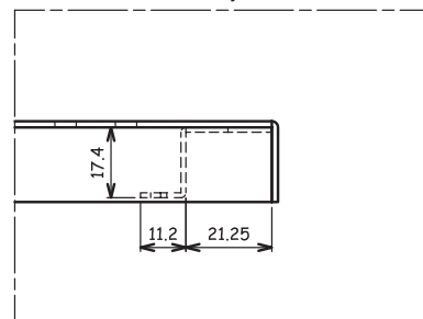
Detalj Y
